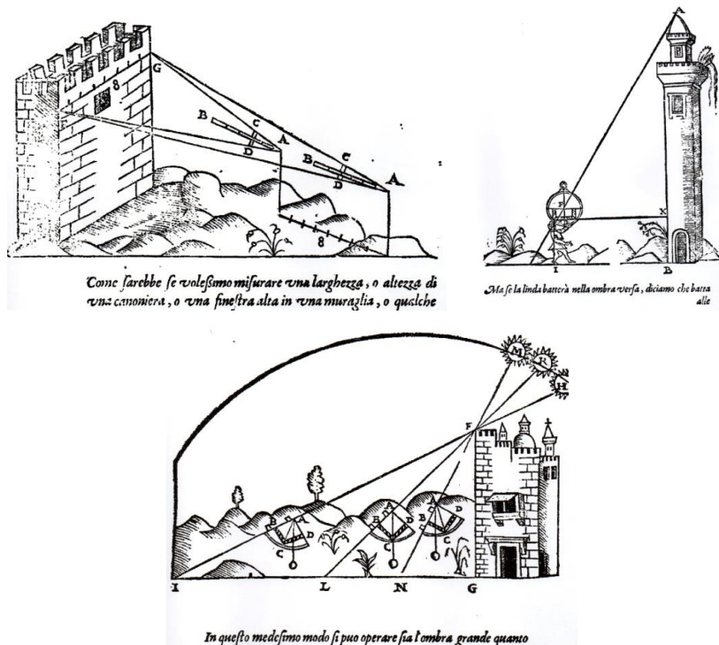
Figura 2: No báculo a medida é dada pelo deslocamento do observador; à direita e embaixo, a medida depende também da altura do observador (BARTOLI, 1564, p. 11v, 23 e 15v).
