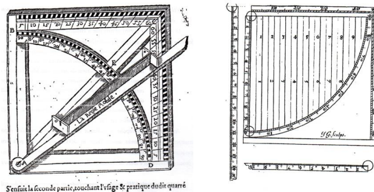
Figura 3: Da esquerda para a direita, o quadrante geométrico de Oroncio Fineo (1556, p. 3v) e o setor trigonal de John Chatfeild (1650, p. 1)
