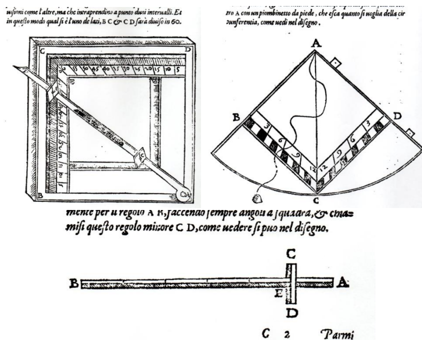
Figura 1: Da esquerda para a direita temos o quadrante geométrico e o quadrante num quarto de círculo e, abaixo, o báculo (BARTOLI, 1564, p. 3r, 8r e 10r)
